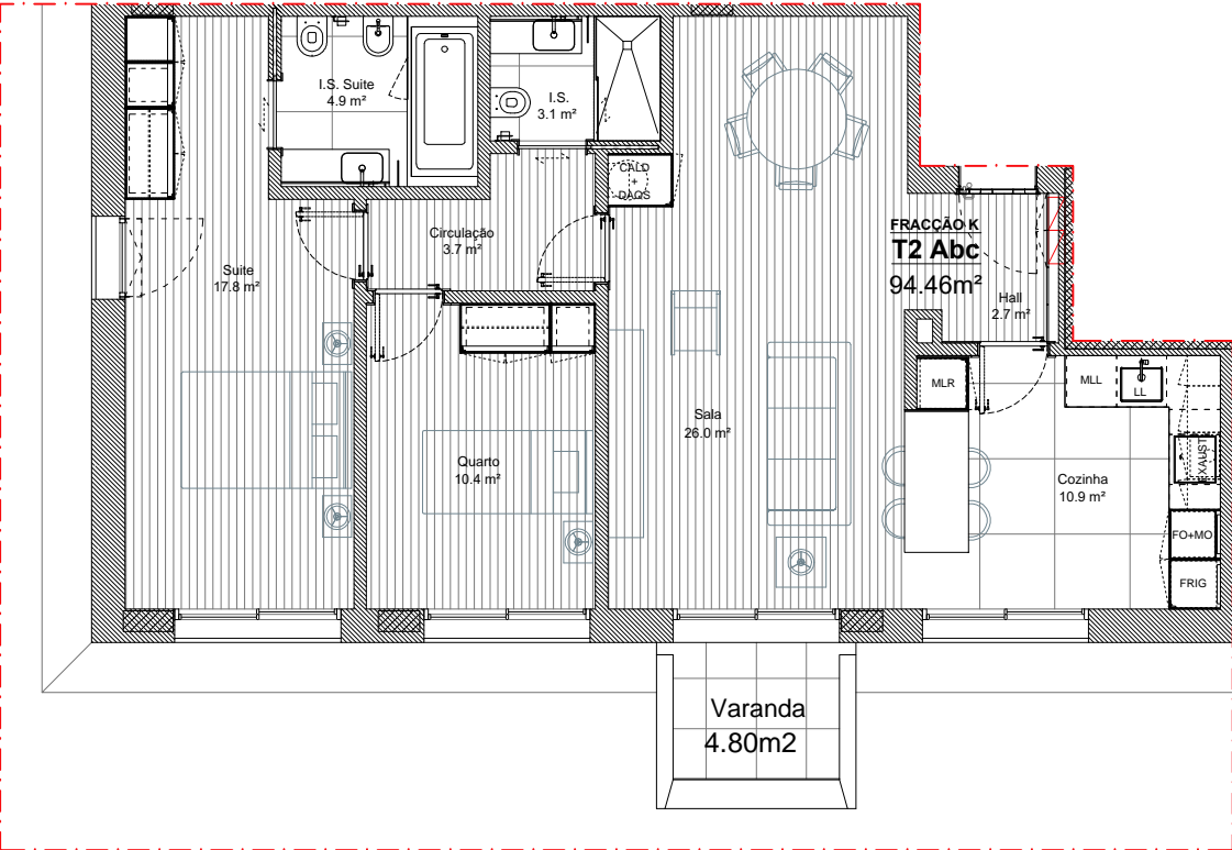
PLANTA 1/100
