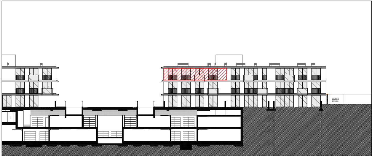
ALÇADO/ CORTE 8 1/500
