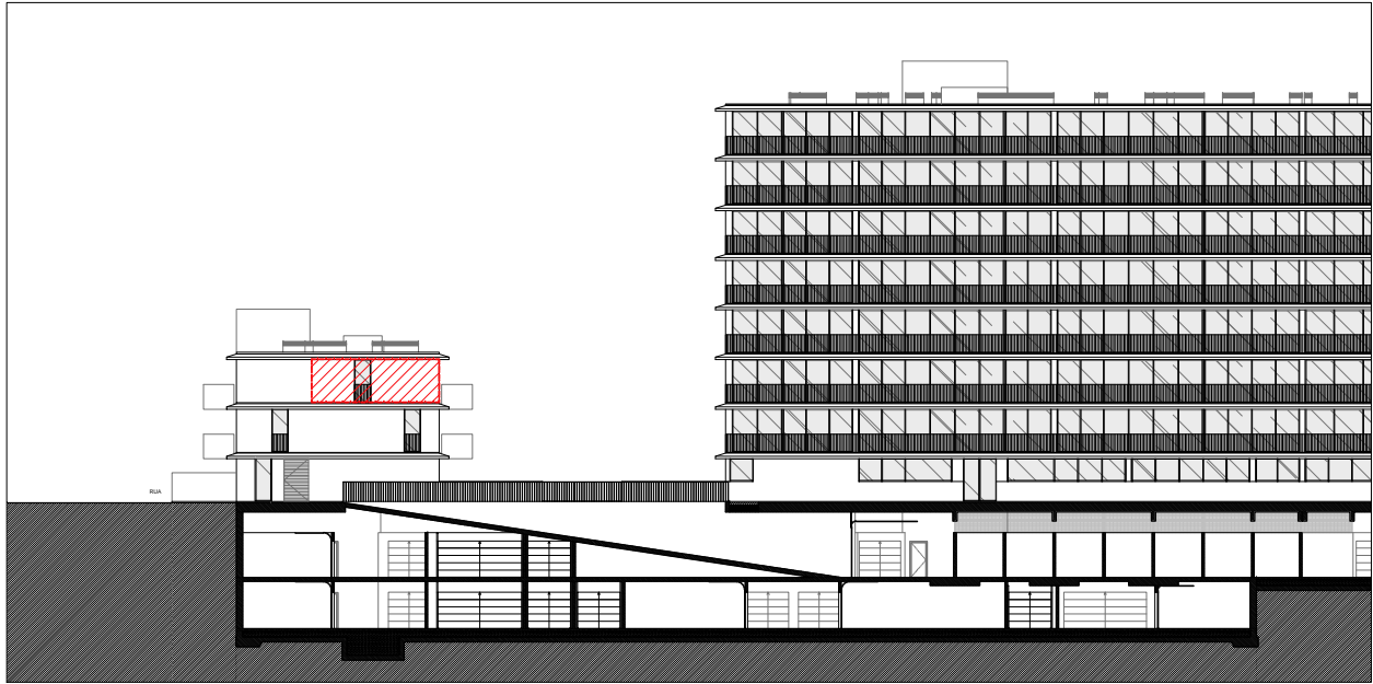
ALÇADO/ CORTE 5 1/500
