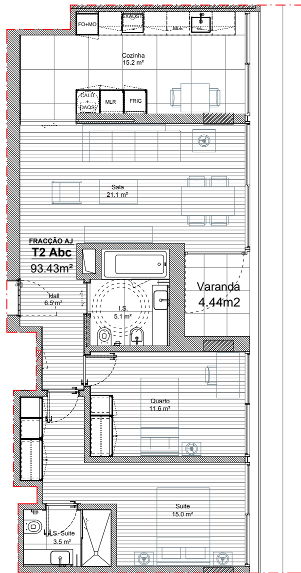
PLANTA 1/100
